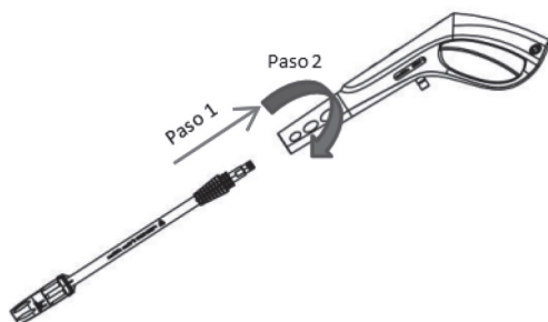
Fig. 5 – Montaje de la lanza
